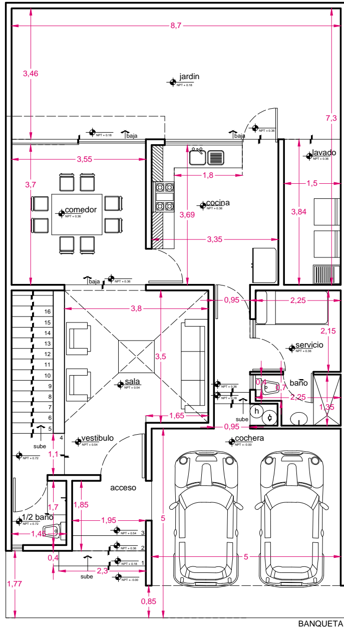
Planta baja Haras Tipo A Sup. Total = 204 m2
