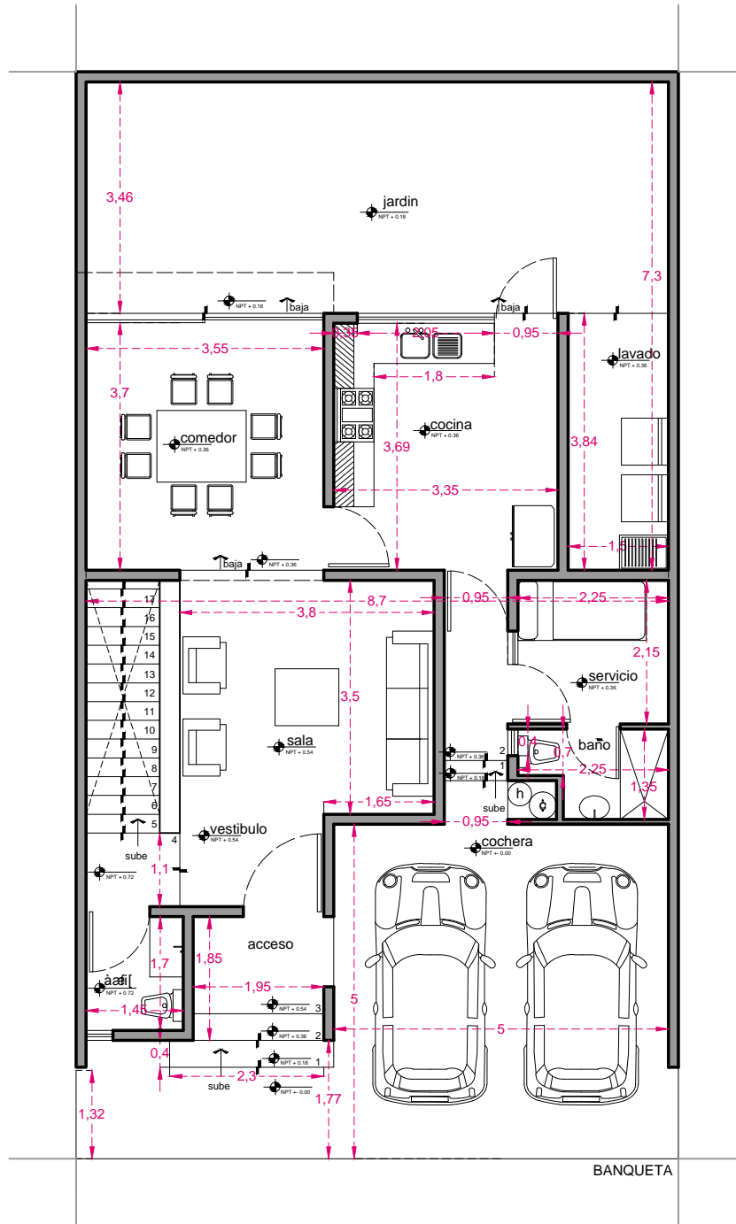
Planta baja Haras Tipo B Sup. Total = 160.65 M2
